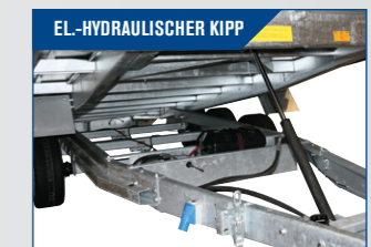
EL.-HYDRAULISCHER KIPP Komplett mit eingebauter Batterie und Ladegerät. Wird mit Fernbedienung mit Kabel geliefert.
