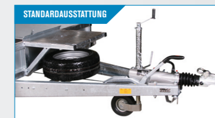
Schaufelablage, Ersatzrad und das Stützrad sind Standard.
