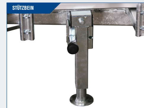
Die kräftige Klappkurbelstütze, sorgt für sicheres und stabiles be- und entladen. 2 Stück als Set, inkl. Handkurbel.
