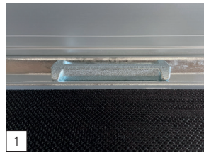
Serienausstattung: vom TÜV zertifiziertes Ladungssicherungssystem von HÄPERT: im Seitenrand integrierte Bindebügel zu je 1000 daN.
