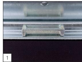
Serienausstattung: Verzurrbügel mit einer Kapazität von 1000 daN in den Boden integriert.
